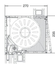
VEKAVARIANT 235 mm Revision vorne mit Insektenschutz
