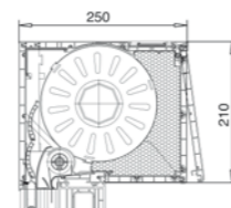
VEKAVARIANT 210 mm Revision vorne mit Insektenschutz
