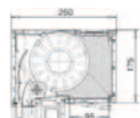
VEKAVARIANT 175 mm Revision unten mit Insektenschutz
